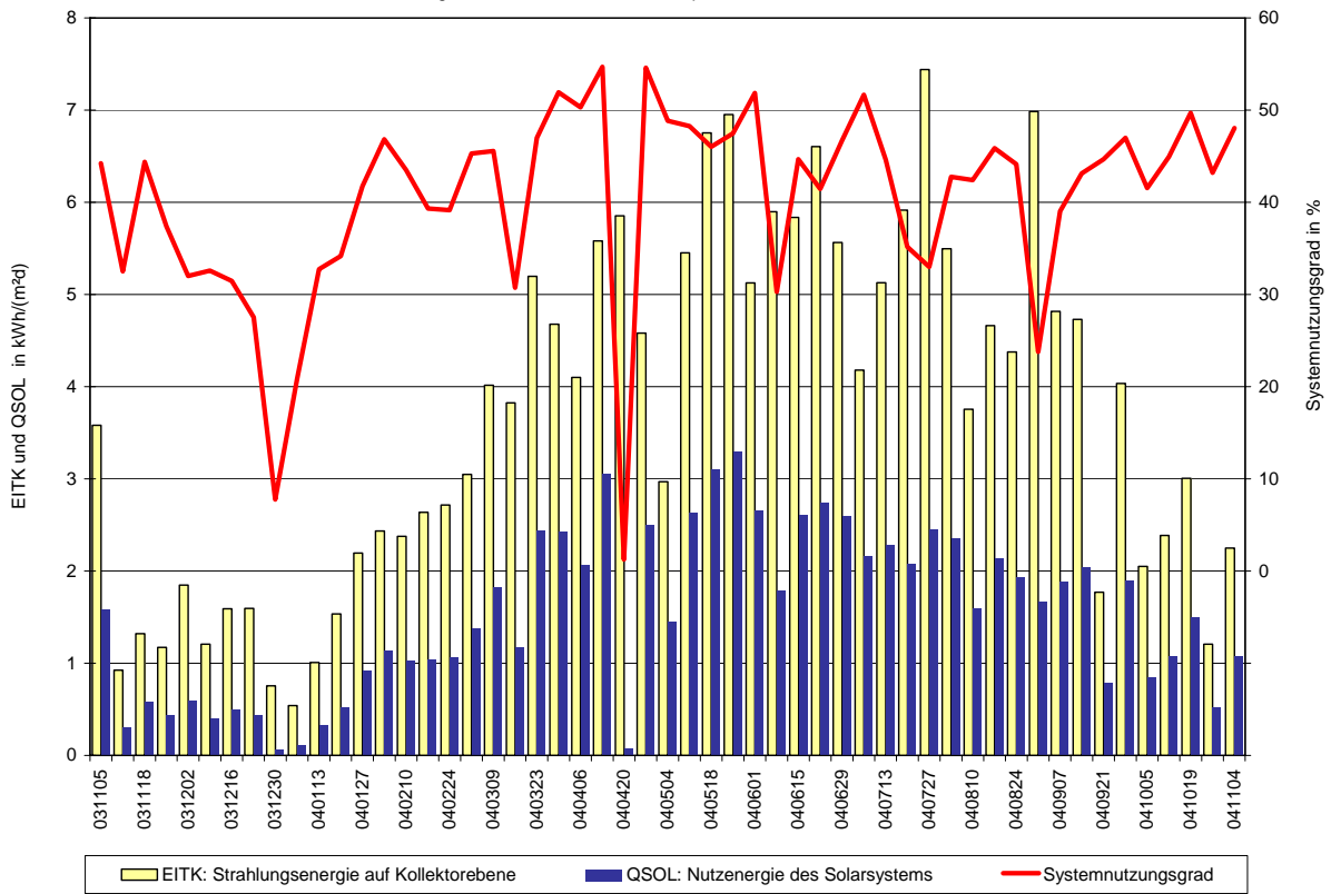
Solaranlage Albtherme Waldbronn: Messperiode 05.11.2003 - 04.11.2004
