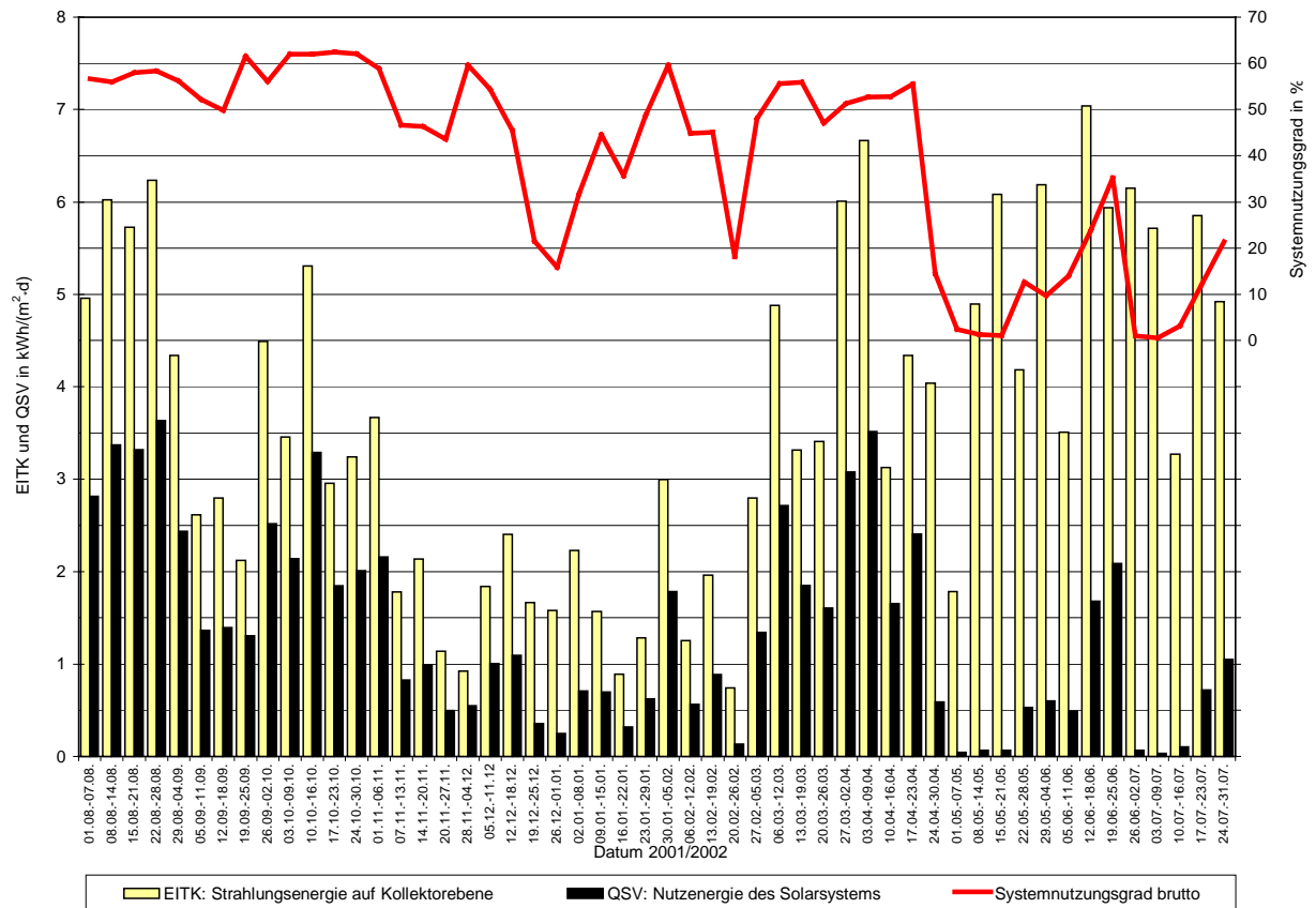
Solaranlage Studentendorf Freiburg-Vauban: Messperiode 01.08.2001 - 31.07.2002
