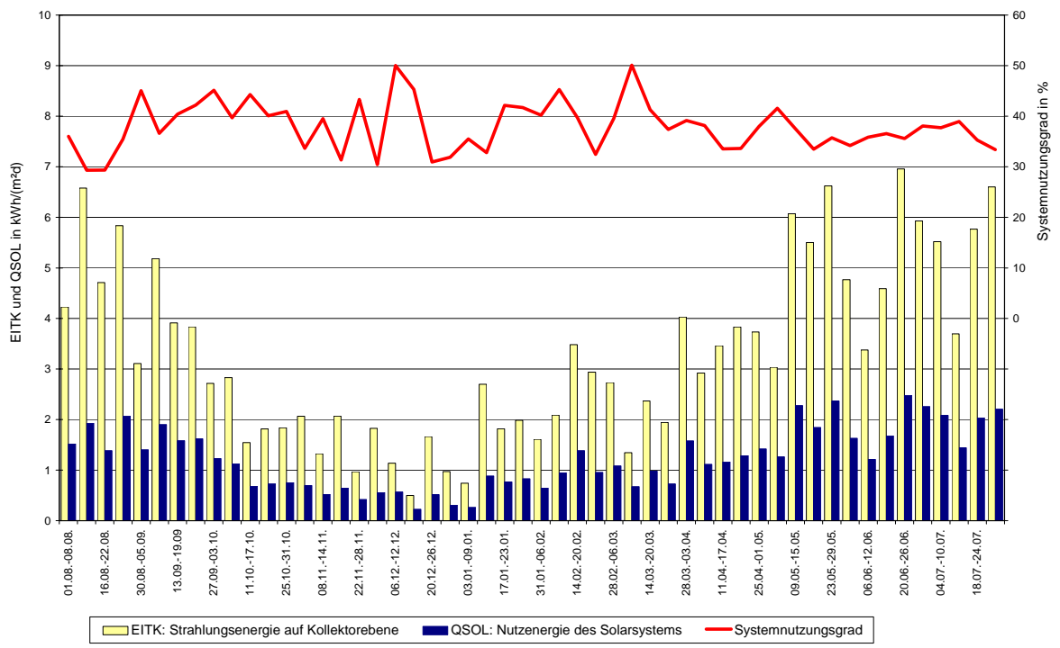
Solaranlage Stadtklinik Baden-Baden: Messperiode 01.08.2000 - 31.07.2001
