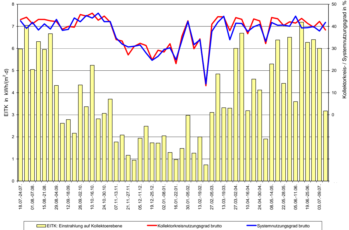
Solaranlage Wohngebäude Wilmersdorfer Str. Freiburg: Messperiode 18.07.2001 - 17.07.2002
