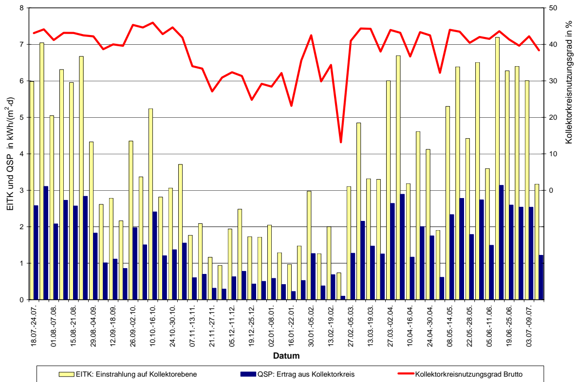
Solaranlage Wohngebäude Wilmersdorfer Str. Freiburg: Messperiode 18.07.2001 - 17.07.2002
