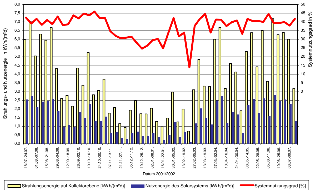
Solaranlage Wohngebäude Wilmersdorfer Str. Freiburg: Messperiode 18.07.2001 - 17.07.2002
