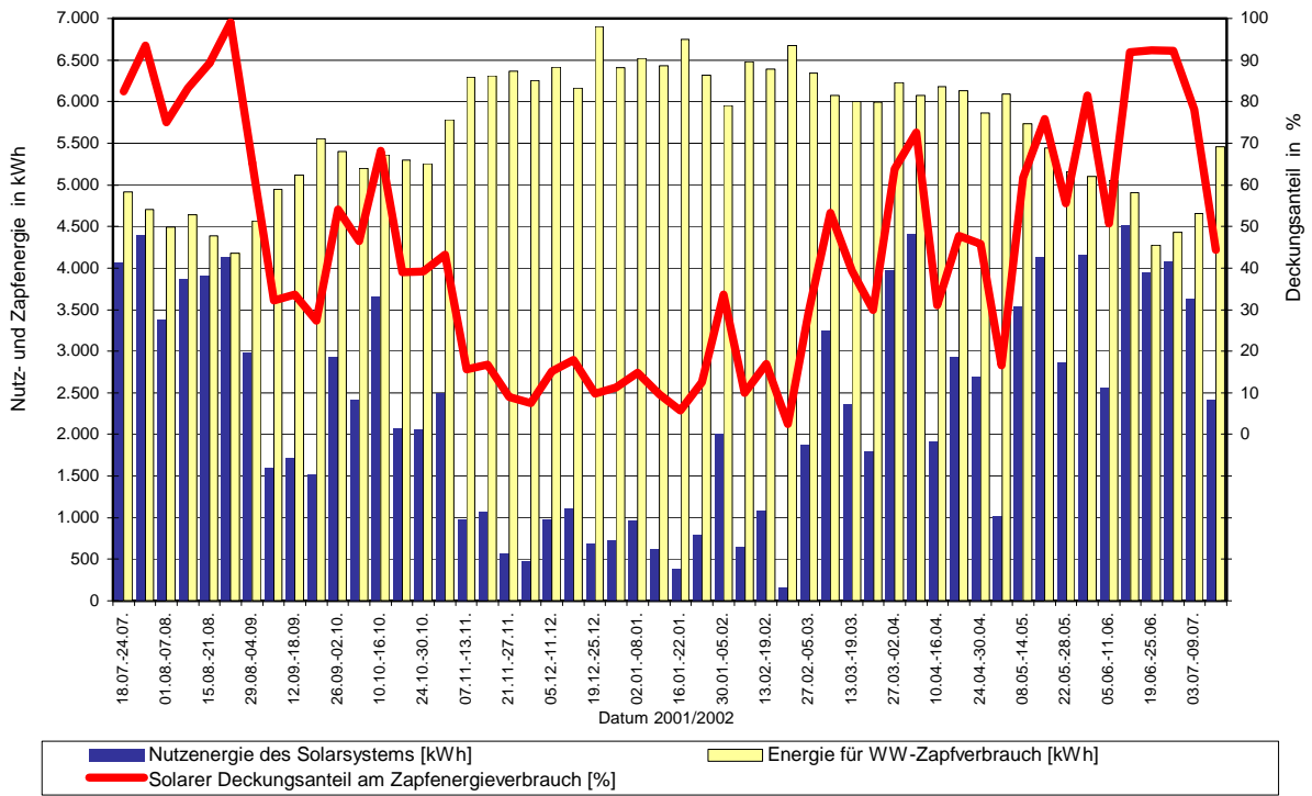
Solaranlage Wohngebäude Wilmersdorfer Str. Freiburg: Messperiode 18.07.2001 - 17.07.2002
