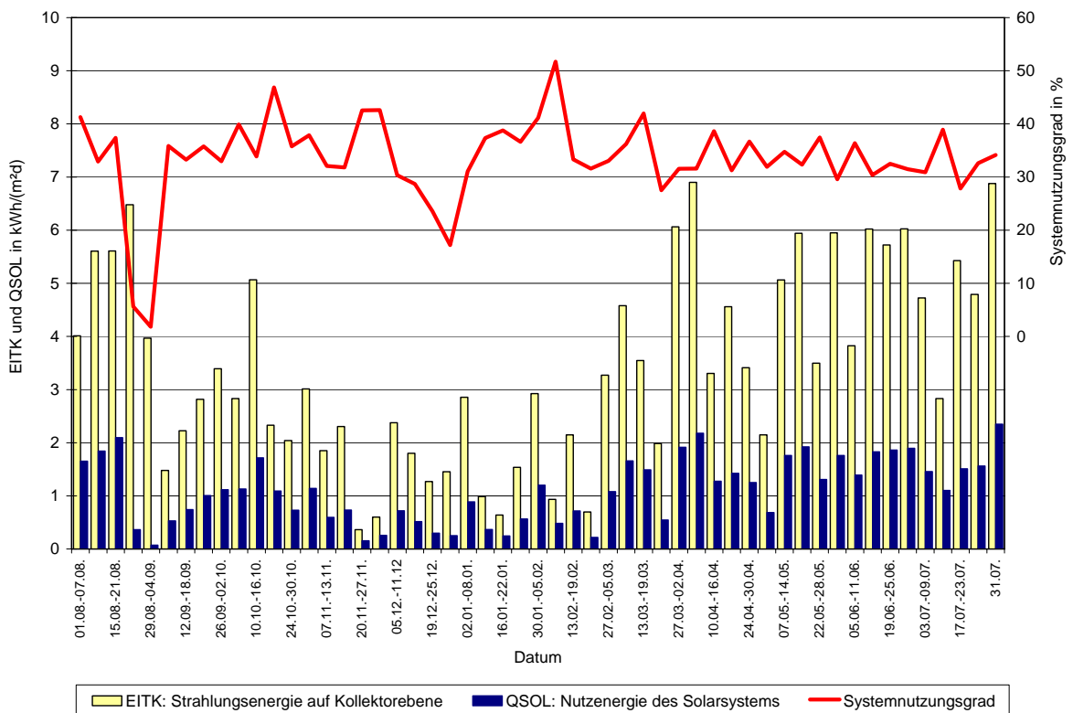
Solaranlage Stadtklinik Baden-Baden: Messperiode 01.08.2001 - 31.07.2002
