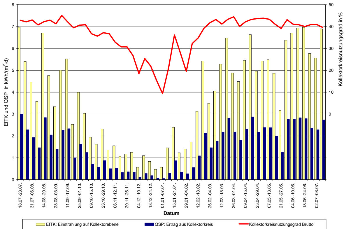
Solaranlage Wohngebäude Wilmersdorfer Str. Freiburg: Messperiode 18.07.2002 - 17.07.2003
