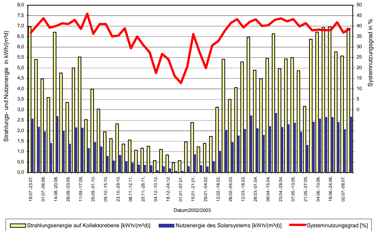
Solaranlage Wohngebäude Wilmersdorfer Str. Freiburg: Messperiode 18.07.2002 - 17.07.2003
