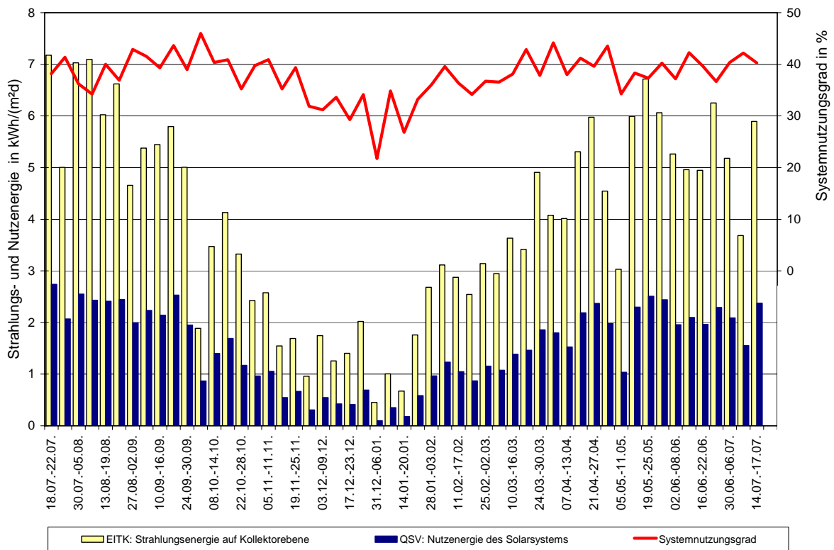
Solaranlage Wohngebäude Wilmersdorfer Str. Freiburg: Messperiode 18.07.2003 - 17.07.2004
