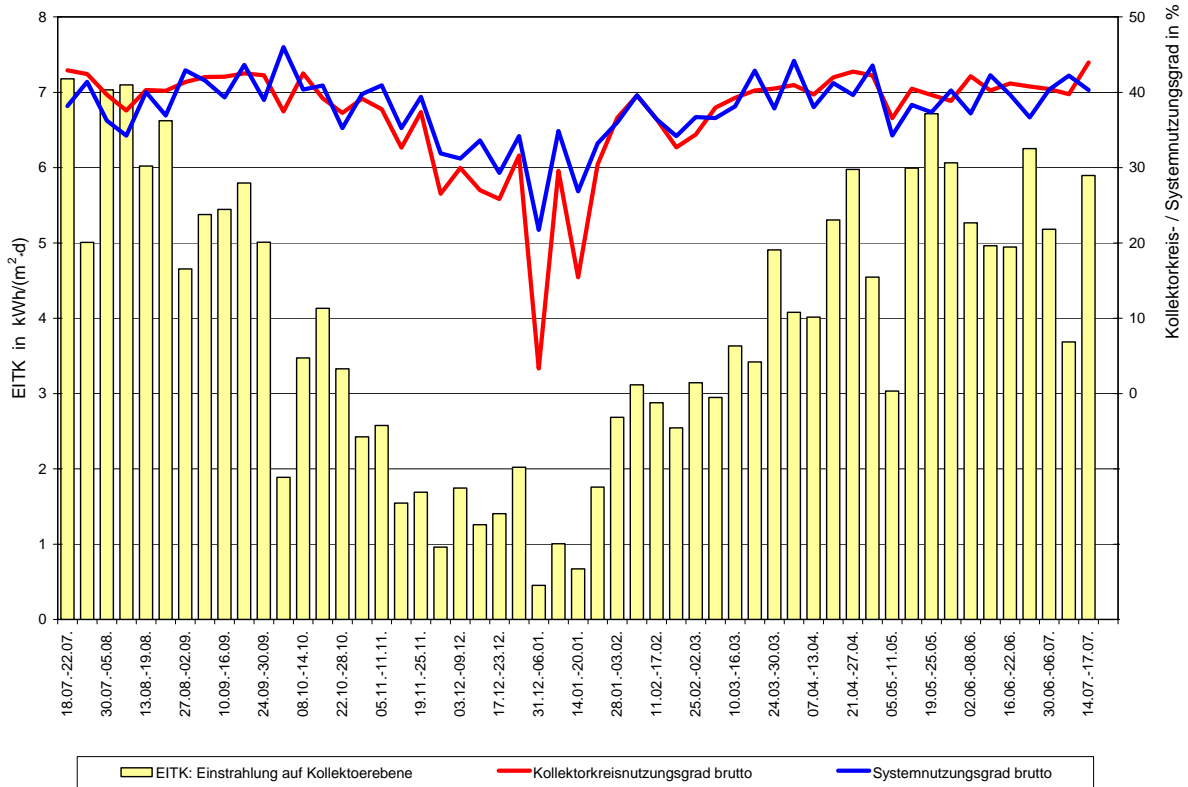
Solaranlage Wohngebäude Wilmersdorfer Str. Freiburg: Messperiode 18.07.2003 - 17.07.2004
